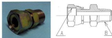
アダプター ORD
