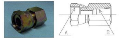
アダプター ORZ
